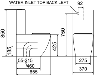
SLIM TOILET SUITE
