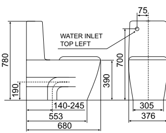
ACACIA EVOLUTION TOILET SUITE
