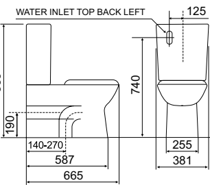
LINFA TOILET SUITE
