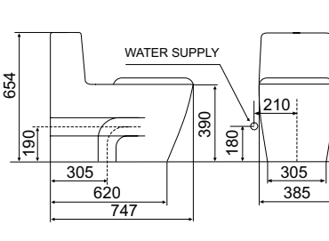
ACACIA EVOLUTION TOILET SUITE
