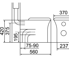
SLIM TOILET PAN
