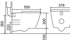
ACACIA EVOLUTION TOILET PAN
