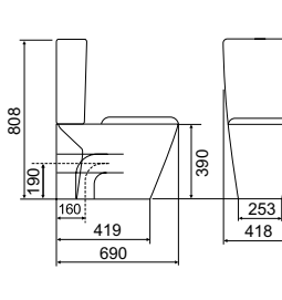
TONIC TOILET SUITE
