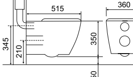
ELLISSE TOILET PAN
