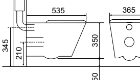
LINFA TOILET PAN
